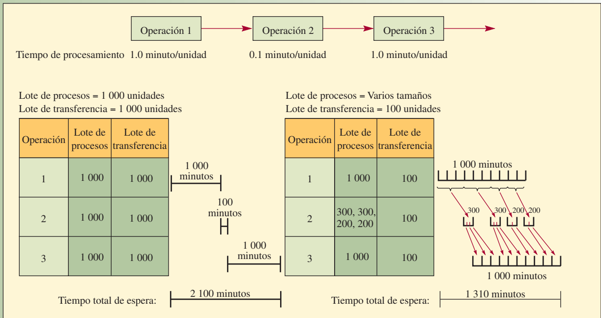
Efecto de cambiar el tamaño del lote de procesos sobre el tiempo de espera de producción en un pedido de trabajo de 1 000 unidades
