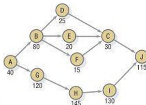
FIGURA 8.14 | Diagrama de precedencia
