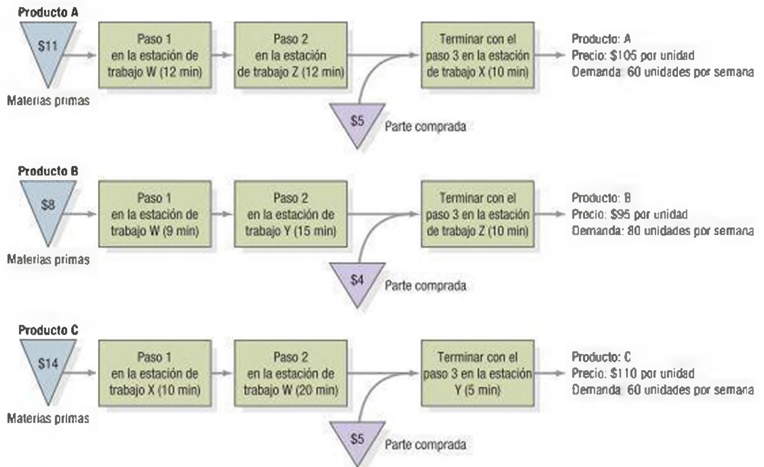
FIGURA 7.11 | Diagrama de flujo para Yosi Perry Industries (YPI)
