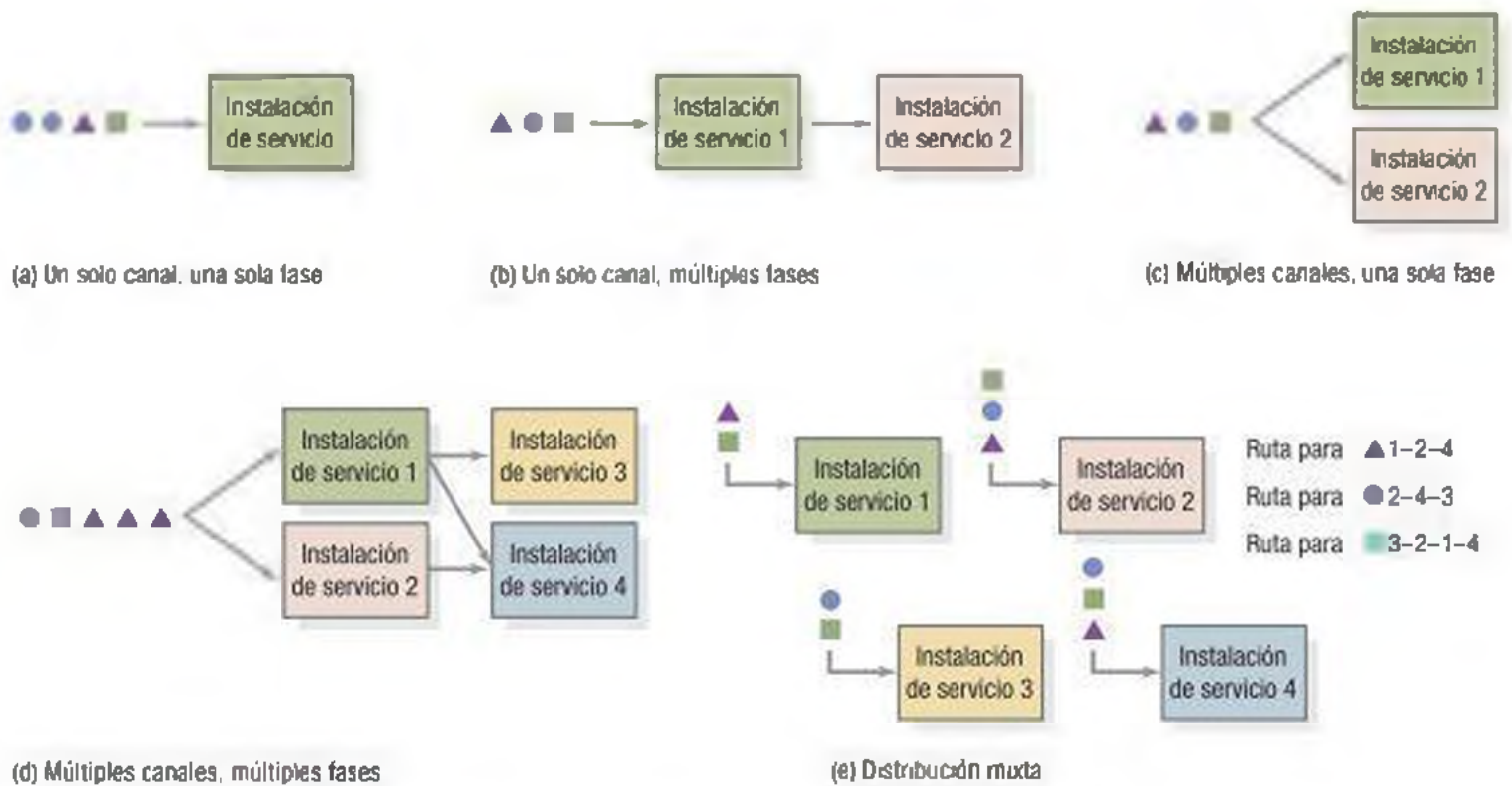
FIGURA C.3 | Ejemplos de distribuciones de instalaciones de servicio
