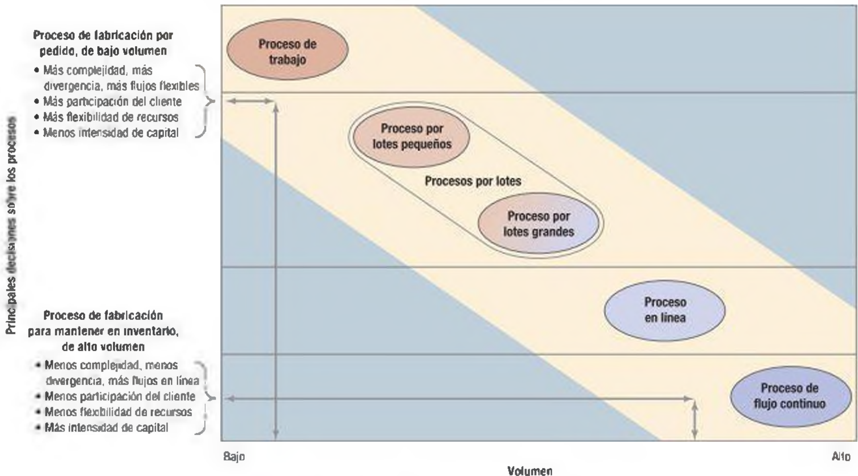
FIGURA 4.10 | Patrones de decisión para procesos de manufactura
