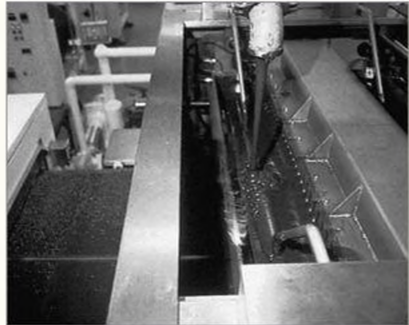
El chocolate caliente se vierte en un tanque de retención en la máquina depositadora que forma las gotas de chocolate.
