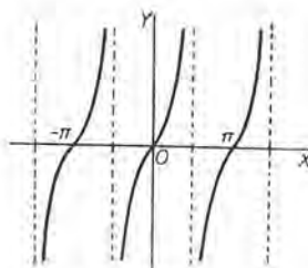
Tangentoide
