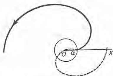
Espiral parabólica
