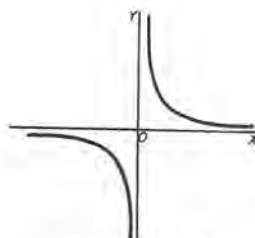
Hipérbola ecuilateral
