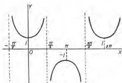
Secantoide
