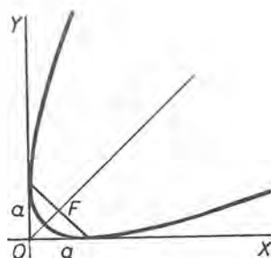
Parábola
