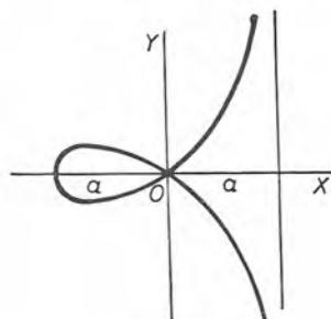
Estrofoide
