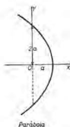
Parábola
