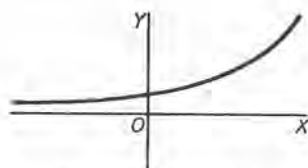
Curva exponencial
