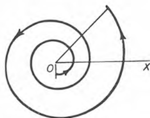
Espirale logarítmica
