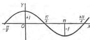
Cosinusoide
