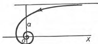
Espirale hiperbólica
